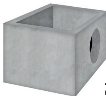
KORYTO BETONOWE Z POKRYWĄ ŻELIWNĄ KL. D400 500x300x300
