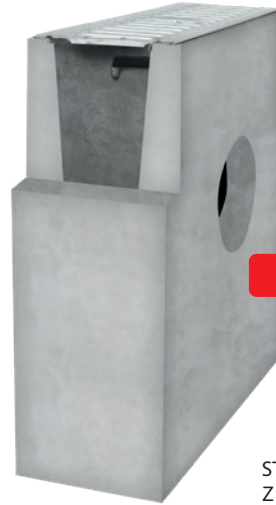
KORYTO BETONOWE Z POKRYWĄ OCYNKOWANĄ KL. A15 1000x130x120
